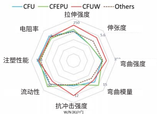
不同涂层碳纤维与树脂改性后的特性对比图
